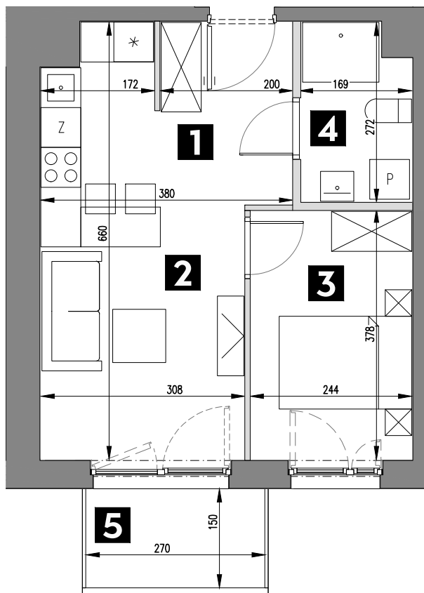
RZUT V PIĘTRA
