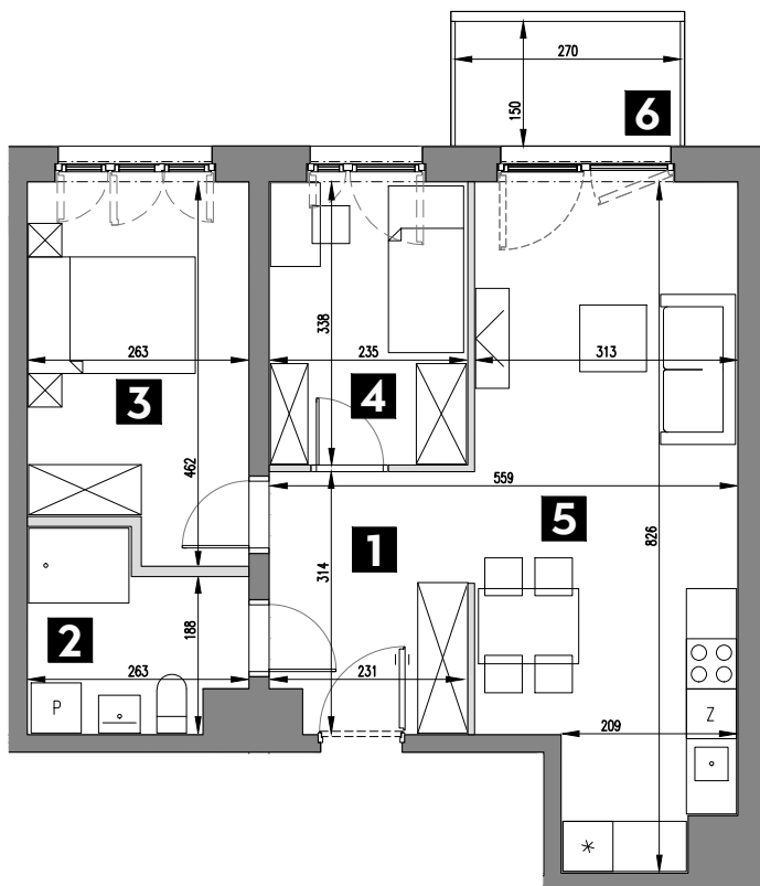
RZUT V PIĘTRA
