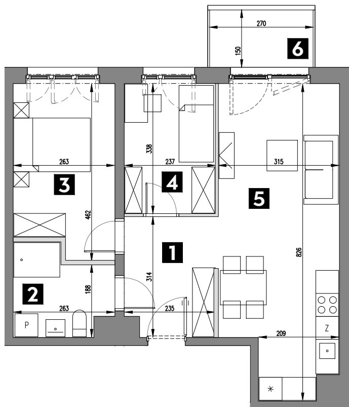
RZUT IV PIĘTRA
