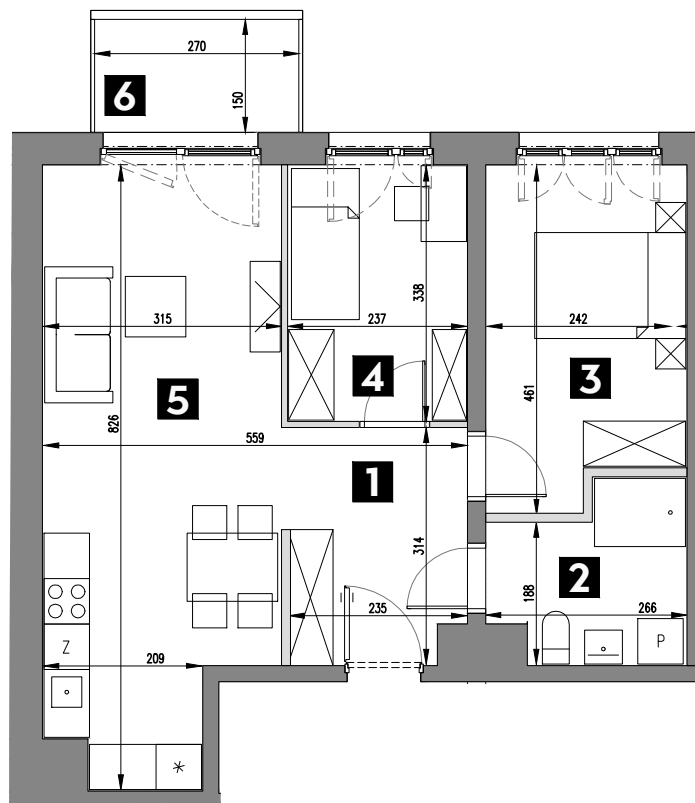
RZUT III PIĘTRA
