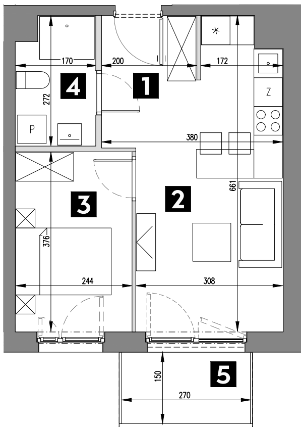
RZUT II PIĘTRA
