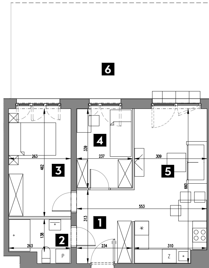
RZUT PARTERU
