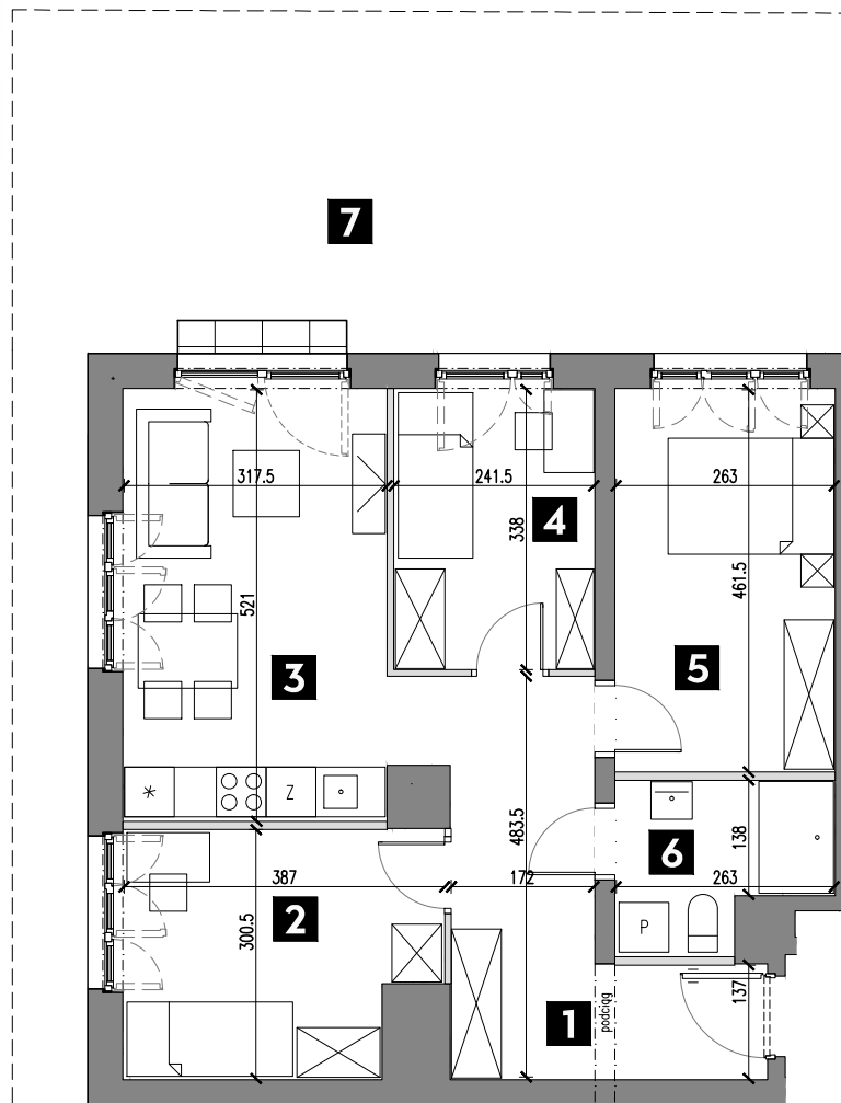
RZUT PARTERU
